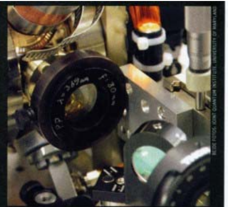
Das Prinzip der quantenmechanischen Datenverarbeitung lässt sich auf dem Labortisch demonstrieren. Die Forscher verwenden einen Laser (das blaue Gerät in der Fotografie links), dessen Strahlen durch mehrere Spiegel bis zu dem Apparat geleitet wird, der die gefangenen Ionen enthält (oben). Der Laser kühlt das Ion – entzieht ihm also seine kinetische Energie –, so dass die Forscher es leicht manipulieren können.
