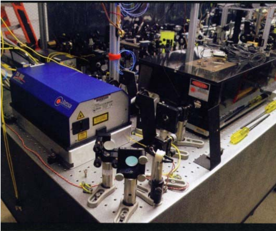
Das Prinzip der quantenmechanischen Datenverarbeitung lässt sich auf dem Labortisch demonstrieren. Die Forscher verwenden einen Laser (das blaue Gerät in der Fotografie links), dessen Strahlen durch mehrere Spiegel bis zu dem Apparat geleitet wird, der die gefangenen Ionen enthält (oben). Der Laser kühlt das Ion – entzieht ihm also seine kinetische Energie –, so dass die Forscher es leicht manipulieren können.
